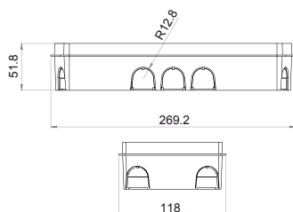
SafeLite Χωνευτή βάση για μπετόν
