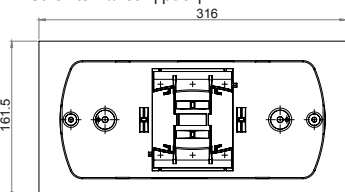
SafeLite Χωνευτή βάση
