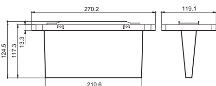
SafeLite Κωνικός διαχυτήρας
