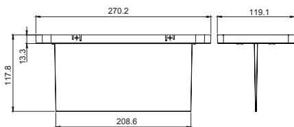
SafeLite Πινακίδα σήματος εξόδου
